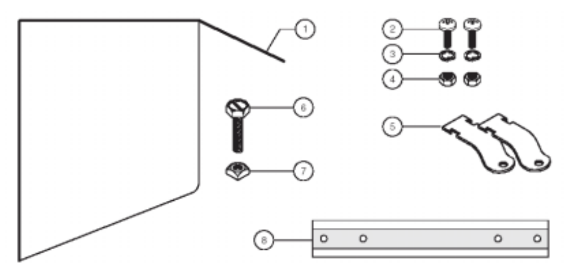
图 3-6 遮阳罩套件
