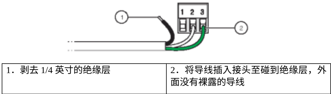
图 3-13 正确的导线制作及插入
