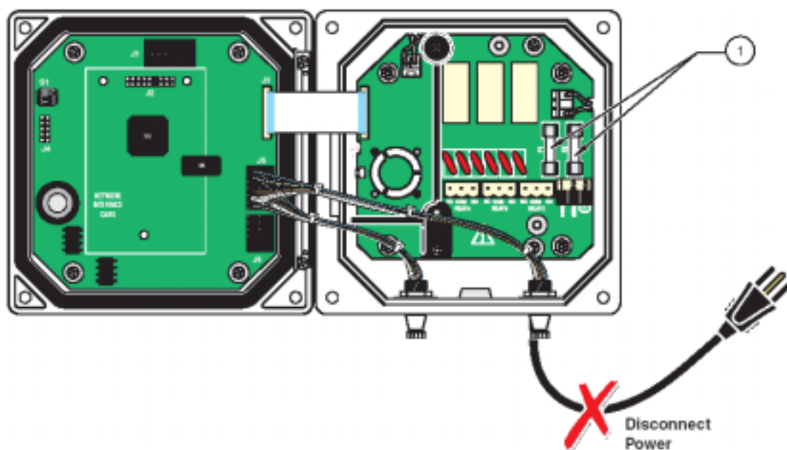
图 4-22 保险丝更换
