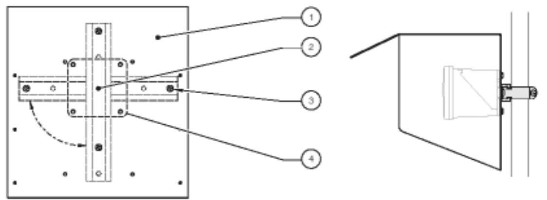
图 3-7 在遮阳罩下安装控制器
